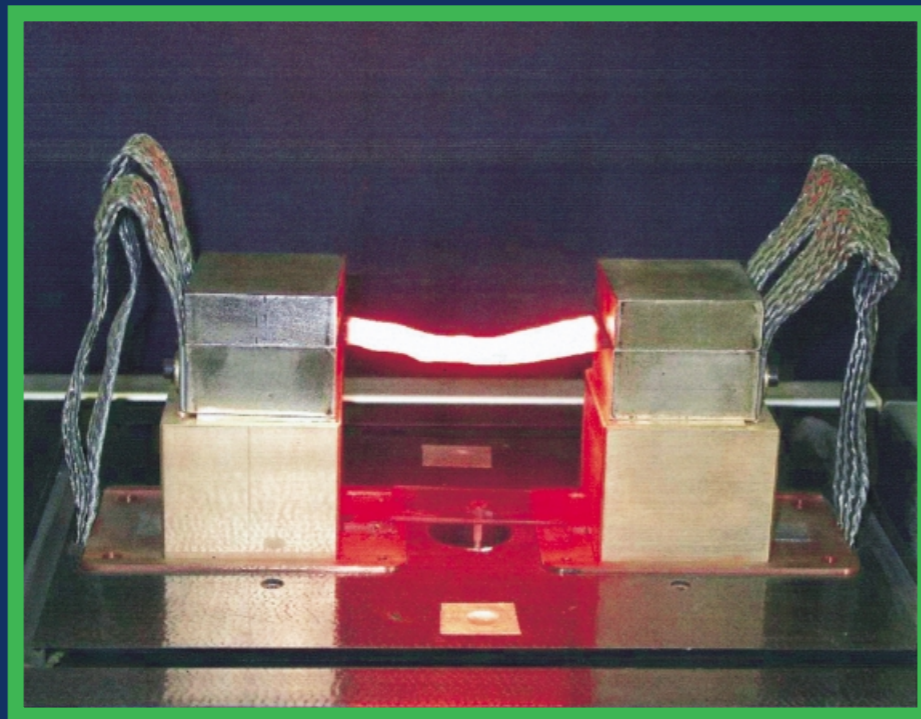
"Reattore a lamina per la pirolisi di combustibili solidi e liquidi"
